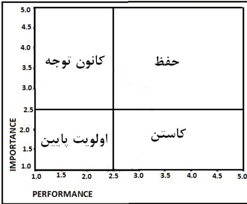
شکل ۲. ماتریس IPA
